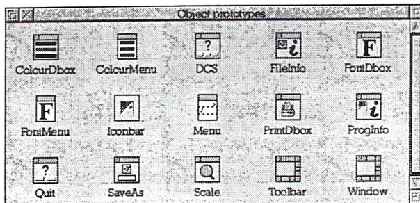
Prototype objecten zijn vrijelijk te gebruiken in de resource editor.
